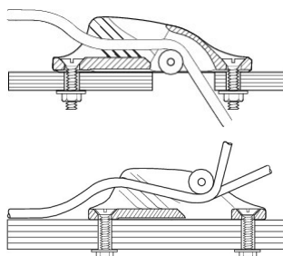
CL270, CL270AN
